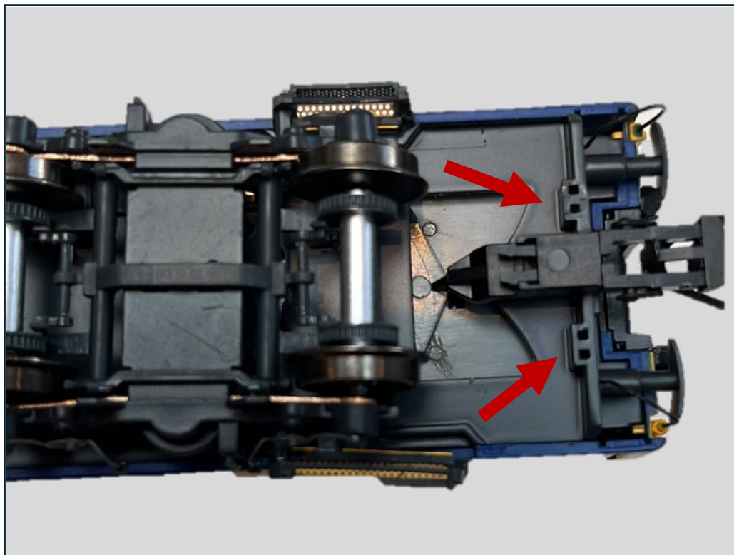
Foto 1: Onderzijde van het rijtuig aan de kant zonder biobak .
